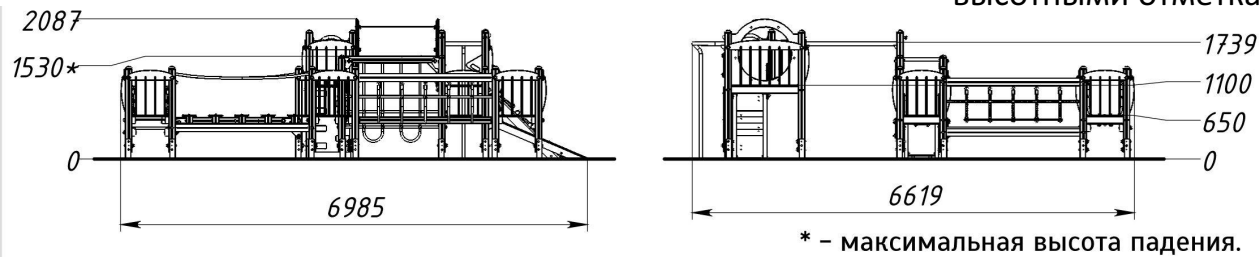
Фасады с обозначенными высотными отметками
